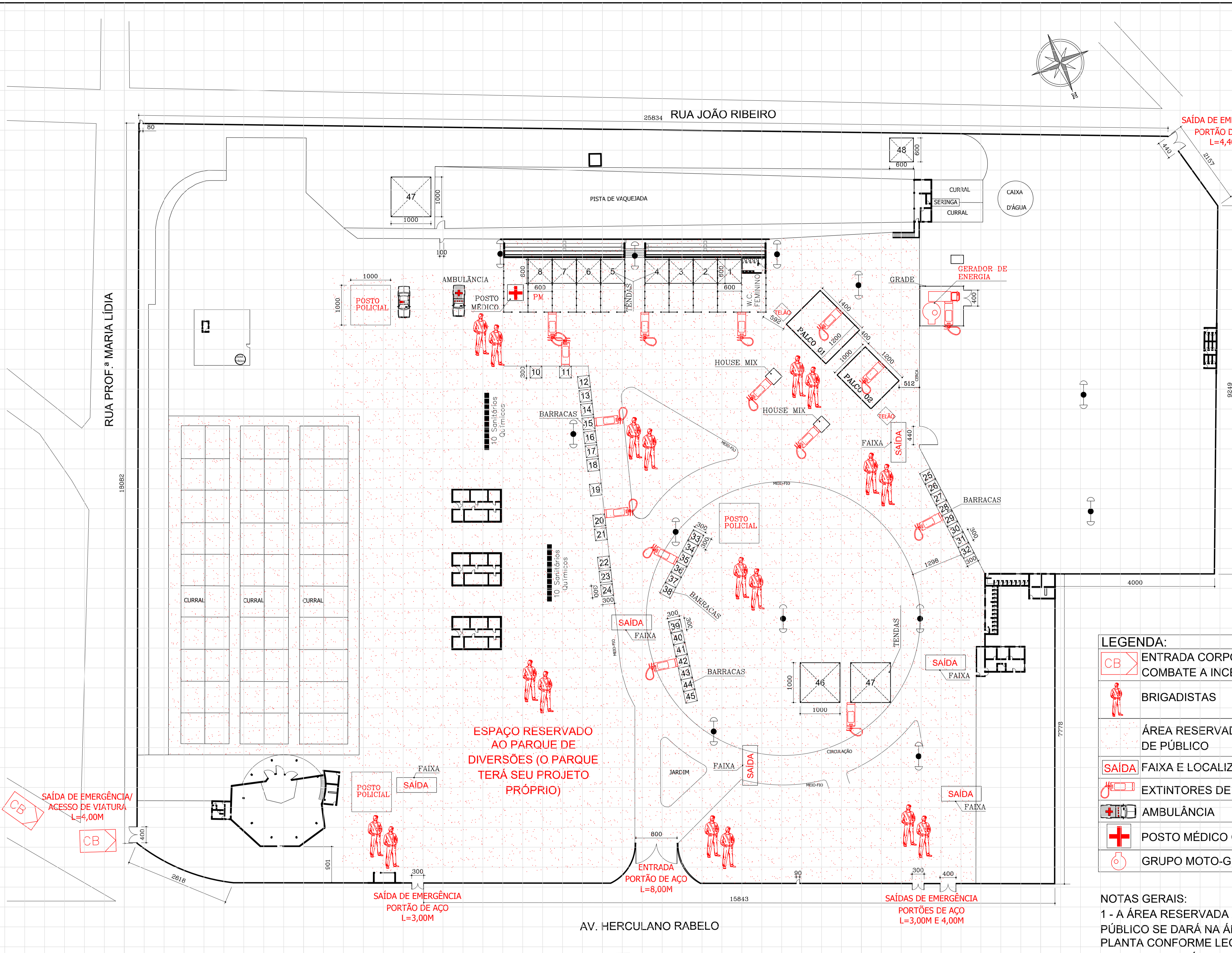
PLANTA DE RISCO ESC.: 1/500
